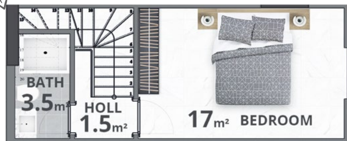
DUPLEX LOWER FLOOR PLAN ПЛАН ДУПЛЕКСНОГО НИЖНЕГО ЭТАЖА
